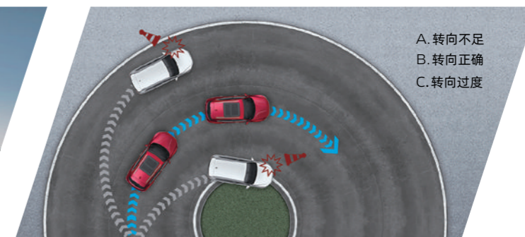
TCS / EDS / ESC / CBC 牵引力控制系统、电子差速锁、车身动态控制系统、弯道制动控制
