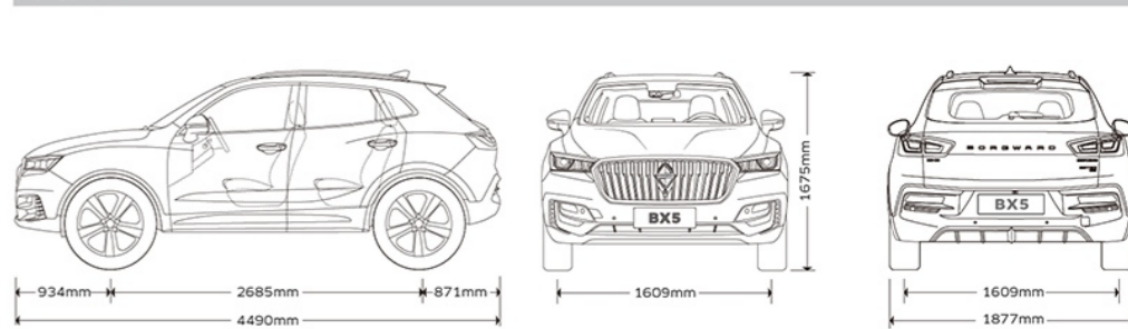
车身尺寸
