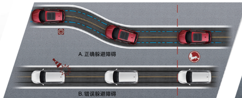
ABS / DTC / BLF / EBP 防抱死制动系统、拖滞力矩控系统、制动灯闪烁、电子预制动
